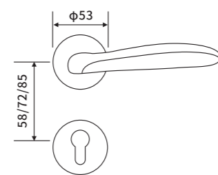
产品尺寸图 Product dimensions
