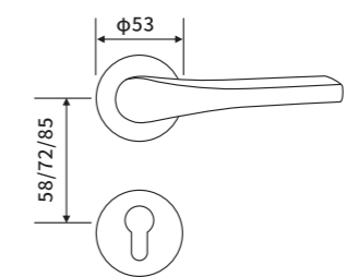
产品尺寸图 Product dimensions
